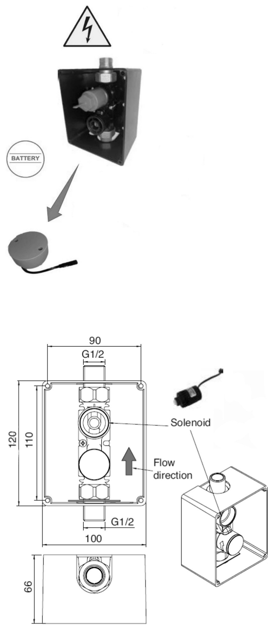
Concealed Box details Détails du boîtier caché
